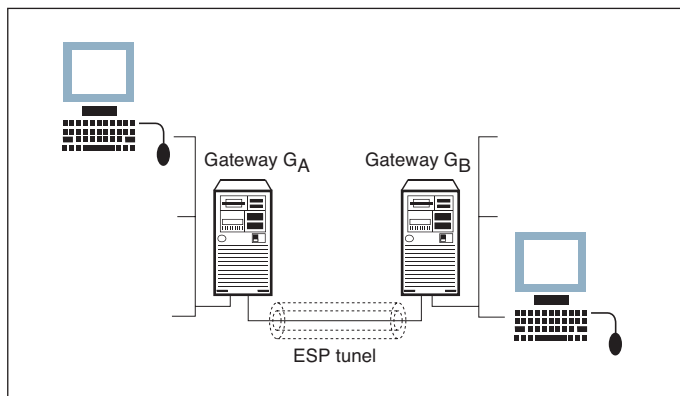
Obr. 1 VPN – šifrované spojení pomocí IPSec (ESP tunel)
